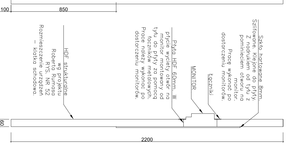
3 Przekrój AA 1:15 @ A3
