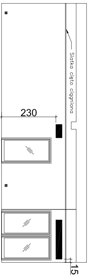
3 Przekrój AA 1:100 @ A3
