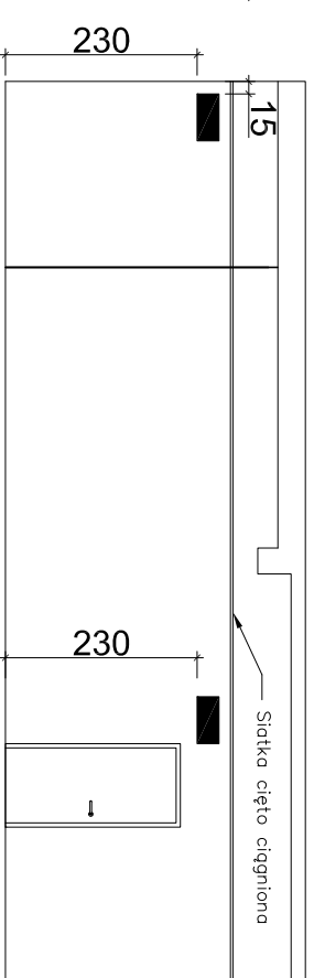
4 Przekrój BB 1:100 @ A3
